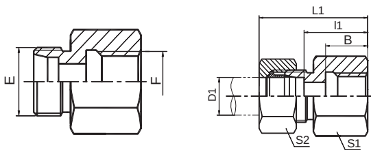
公制内螺纹柱端接头 METRIC FEMALE STUD FITTINGS
