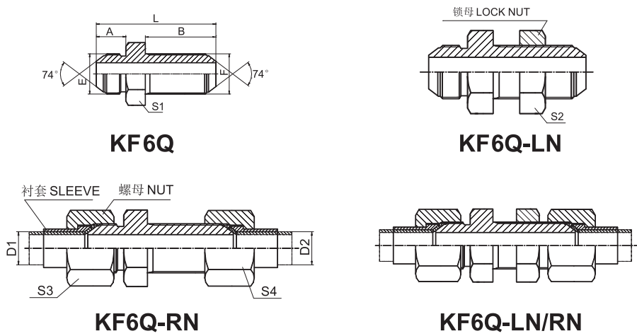
公制外螺纹 74° 外锥过板接头 METRIC MALE 74° CONE BULKHEAD
